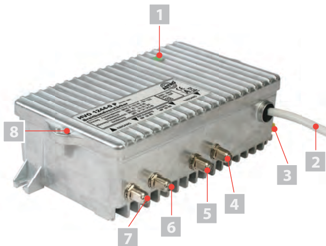
Bild 1: Verstärker HVO 1244-0 P
